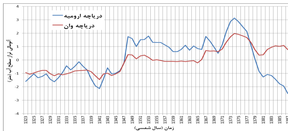
نمودار ۹- سری زمانی آنومالی سالانه تراز دریاچه‌های ارومیه و وان
